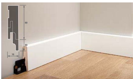
Designfußeiste DFL 60 / DFL 80
