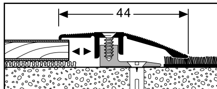
Schraub Ausgleichsprofil 6,5 - 16 / 26 mm
