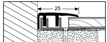
Click Endprofil 6 - 10 / 15 / 20 mm
