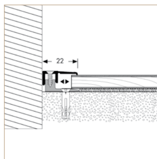
Schraub Endprofilprofil 6,5–16 mm (bis 26 mm mit Lift up Block)
