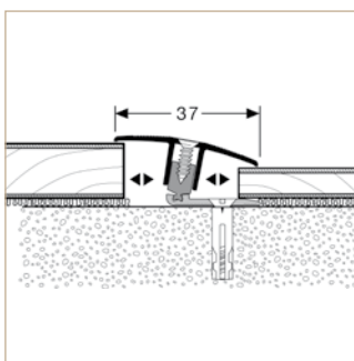
Schraub Übergangsprofil mit Niveaueausgleich bis ca. 5 mm gleich hoch 7–17 mm (bis 27 mm mit Lift up Block) ungleich hoch 3–22 mm (bis 32 mm mit Lift up Block)
