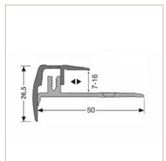
Treppenkantenschiene PF 320 Für Laminat und Parkett, Aluminium eloxiert 7–16 mm
